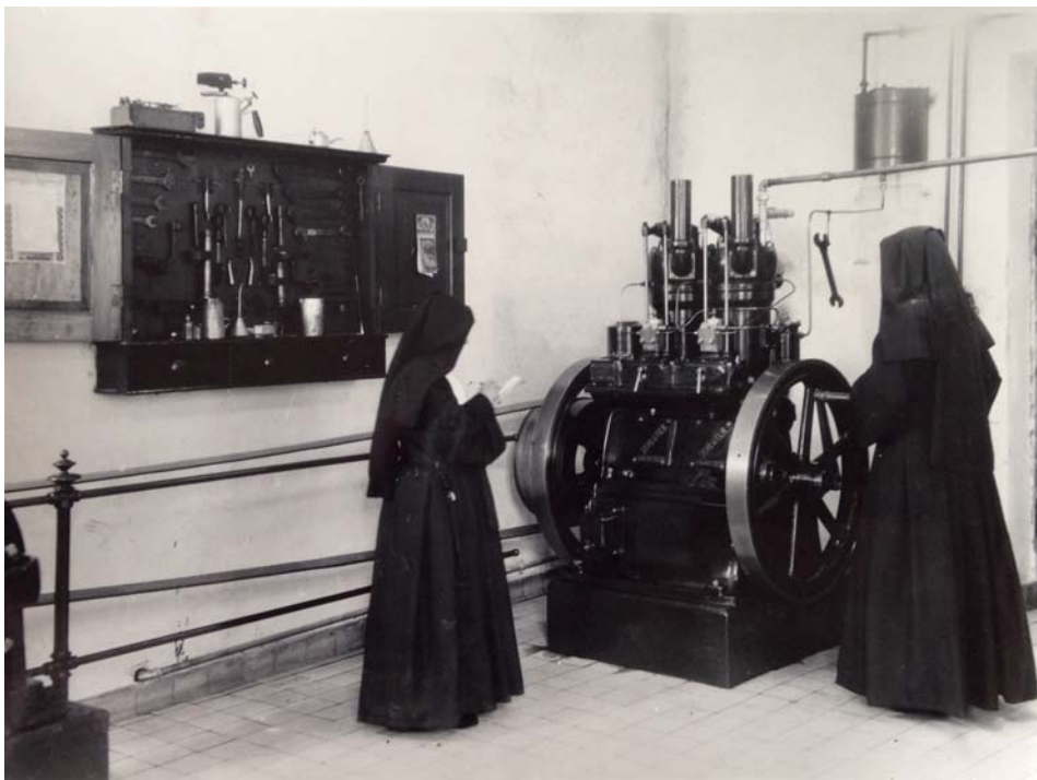
Kraftanlage Kloster Zangberg – Maschinenhaus mit Motor 1926.
